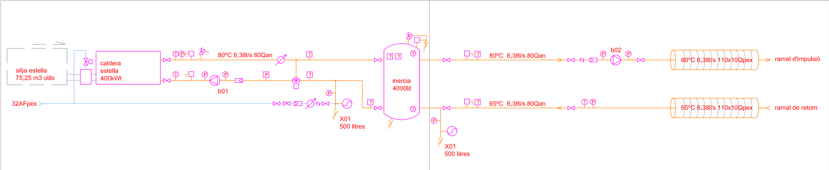
Esquema hidràulic i de fontaneria
