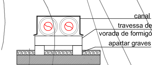
Detall tram coberta edifici. Esc. 1/25
