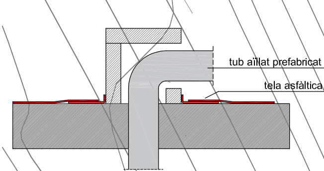
Detall entrada edifici des de coberta. Esc. 1/25
