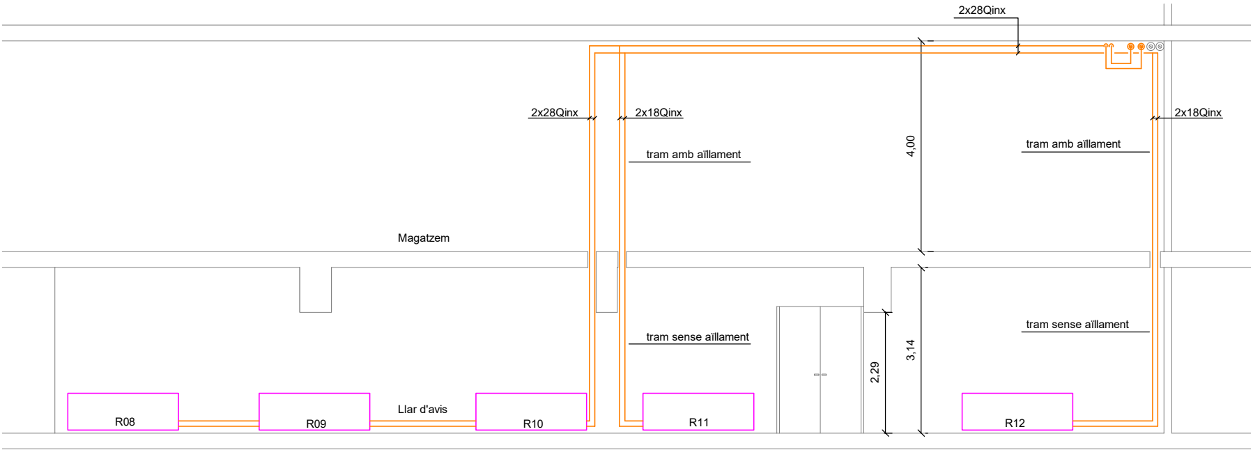
Secció a-a'
