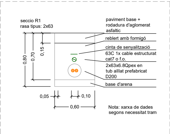
Detall rases Esc: 1/35
