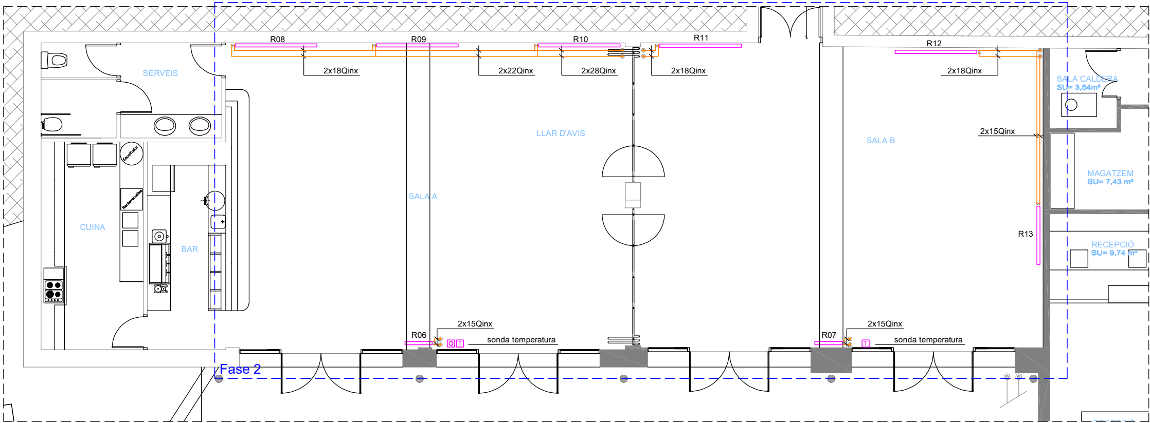
Planta baixa edifici serveis municipals
