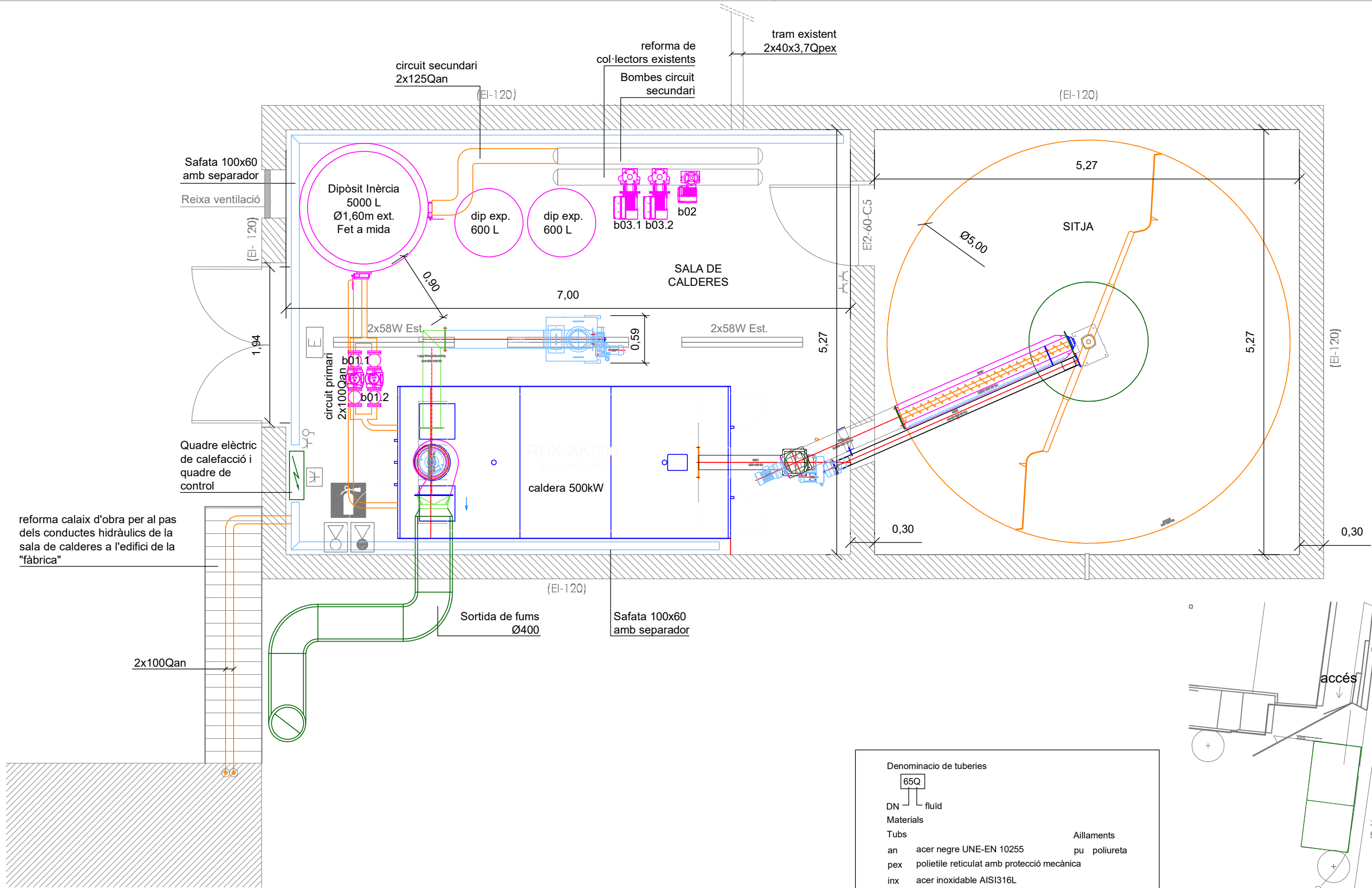
Situació sala de calderes i sitja e: 1/500
