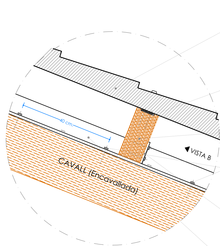
DETALL 3 PROPOSTA - VISTA A ESC. 1/10
