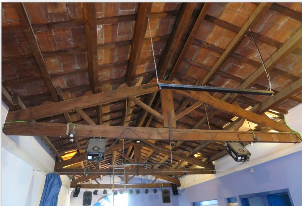
Sostre de la planta baixa (PB). Imatge 602 Vista general
