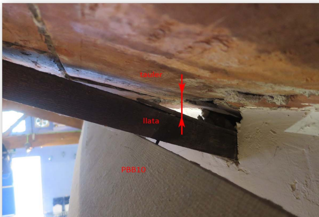
Sostre de la planta baixa (PB). Element PBB10. Imatge 608 Tauler no recolzat sobre les llatas
