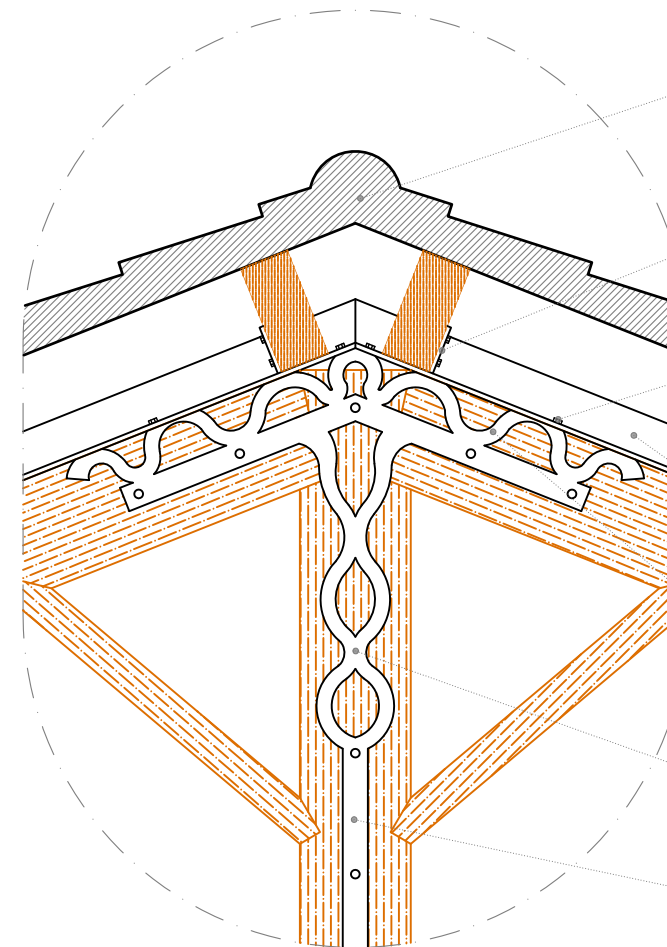
DETALL 2 PROPOSTA ESC. 1/15
