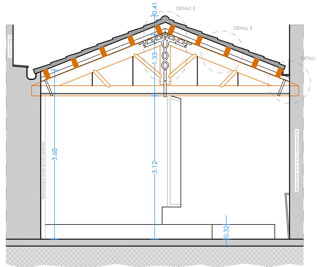
SECCIÓ A-A' PROPOSTA ESC. 1/50
