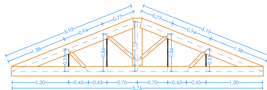
DETALL ENCAVALLADA ESTAT ACTUAL ESC. 1/50
