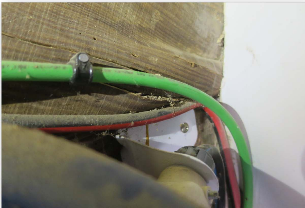
Sostre de la planta baixa (PB). Element PBE3 (encavallada). Imatge 606 Degradació causada per tèrmits subterranis Aixafament del recolzament en l'extrem sud-est
