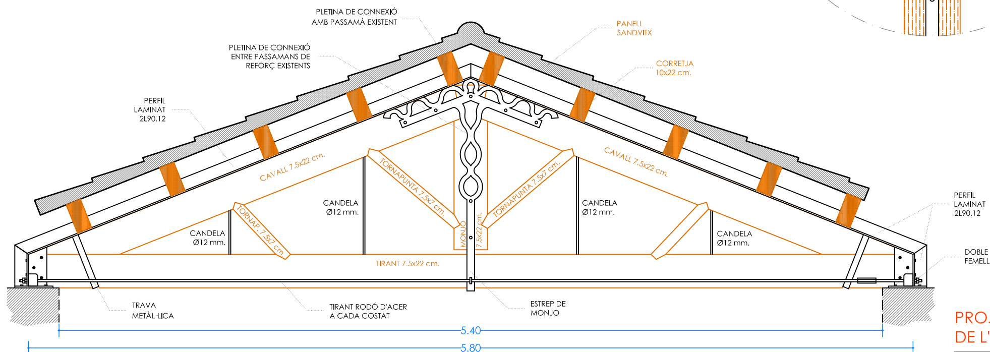
DETALL ESTRUCTURA DE FUSTA PROPOSTA ESC. 1/25
