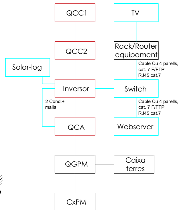
ESQUEMA SINÒPTIC
