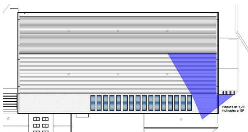
Alternativa amb mòduls a 8° Azimuth i placa de 1,75m
