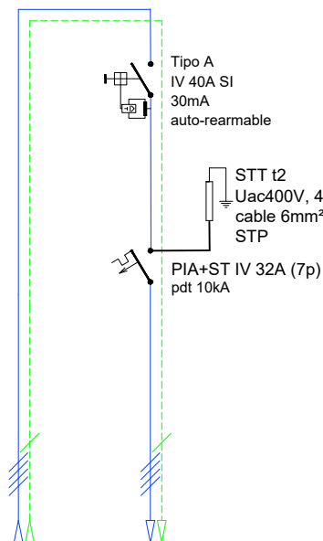
QFCA-QUADRE FOTOV. CA DPI (12) - Dispositius prot. interiors
