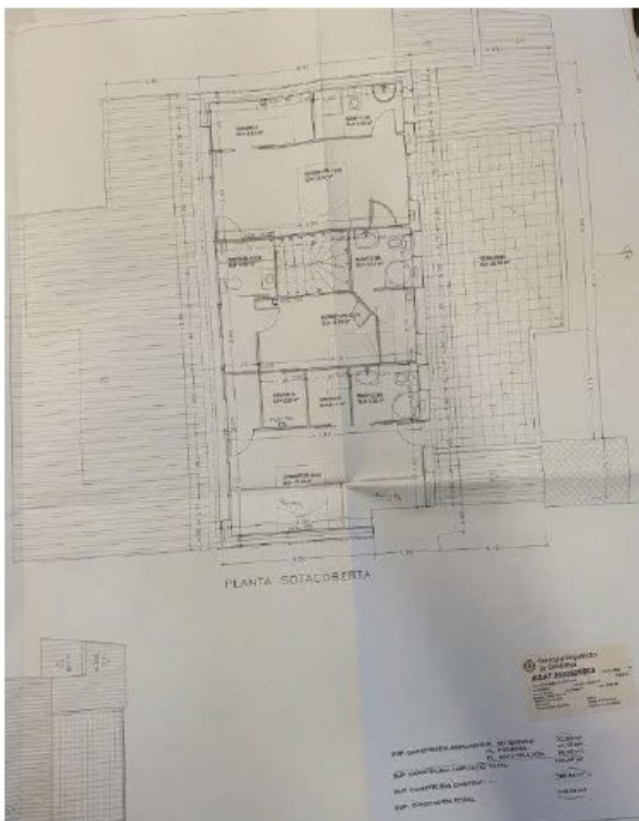
Planta segona
