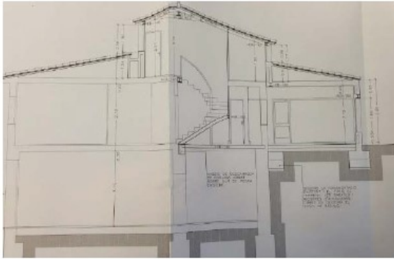
Secció escala
