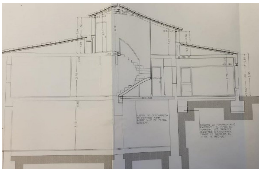
Secció escala
