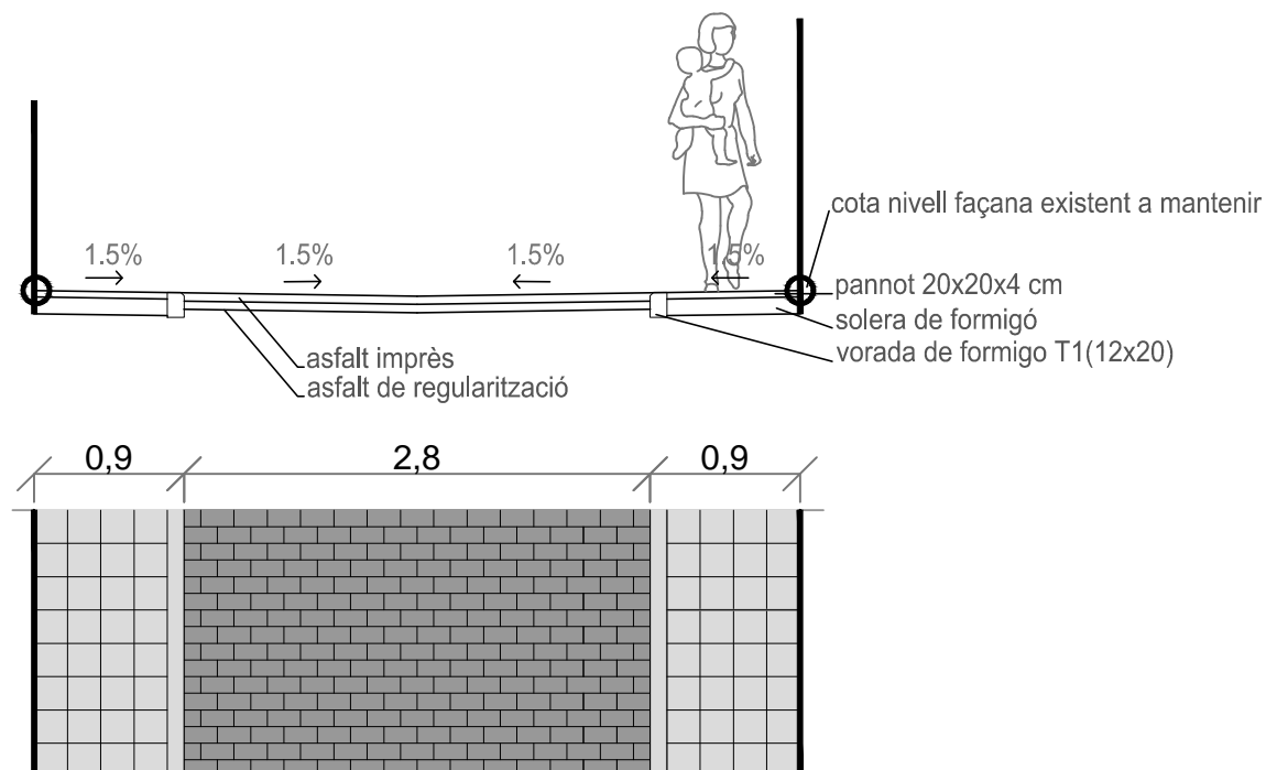
SECCIÓ TIPUS C carrer PAU CASALS
